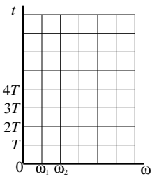
STFT Tiling
