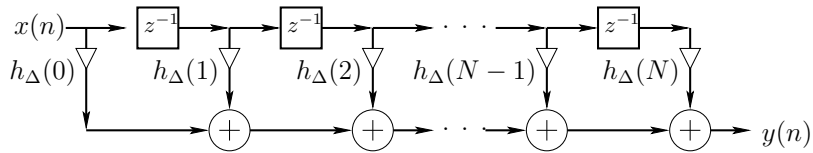
Generic FIR
